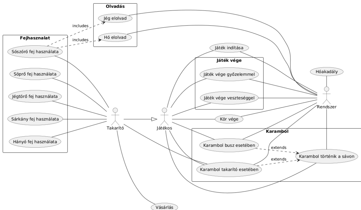
Ábra 1.: A forgatókönyvhöz tartozó use-case diagram
